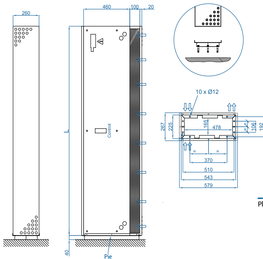
Instalación vertical
