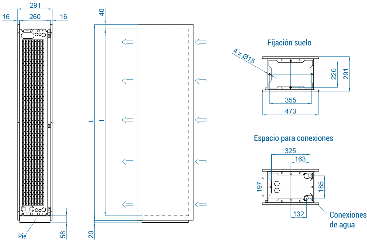
Instalación vertical
