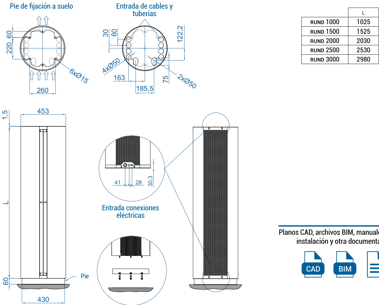
Instalación vertical
