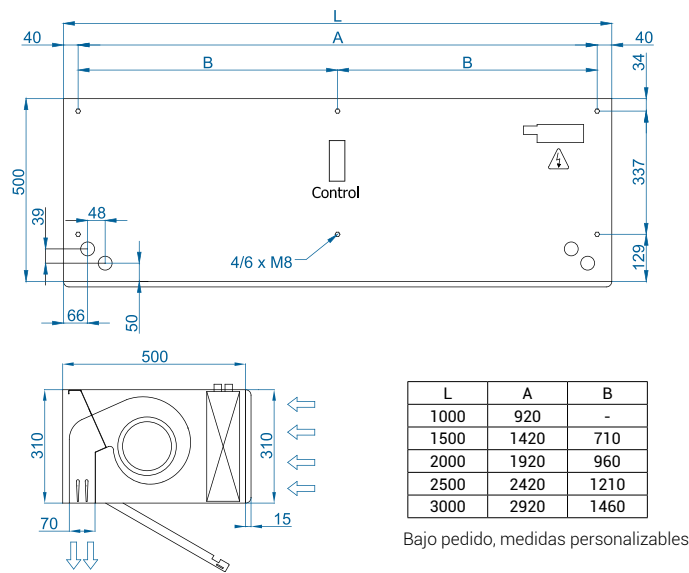
Instalación horizontal
