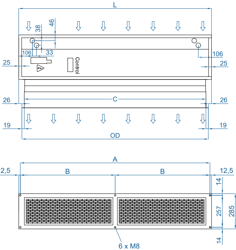
Instalación horizontal
