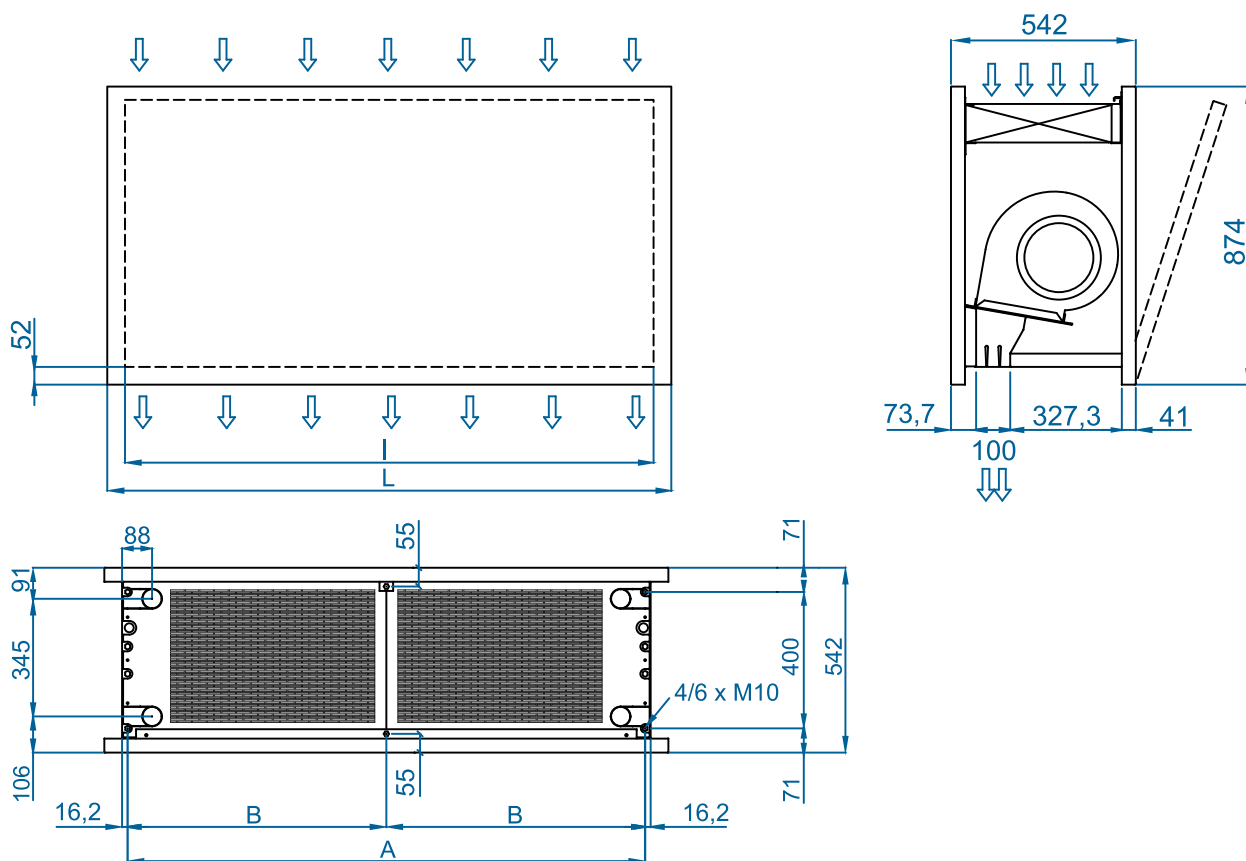
Instalación horizontal
