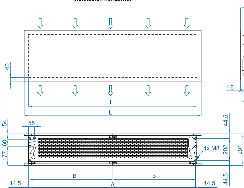
Instalación horizontal
